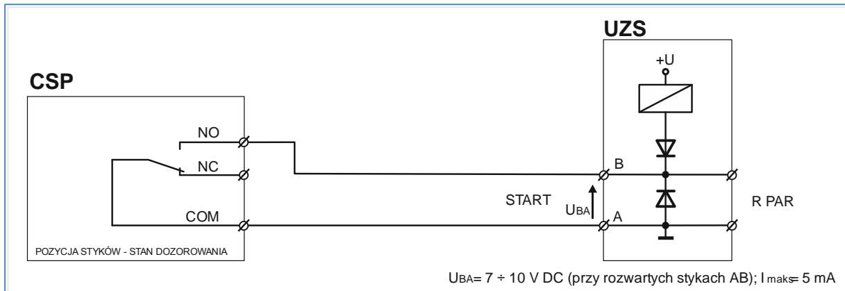
Rys. 14 Sterowanie wyjściem przekaźnikowym bezpotencjałowym (wariant 1).
