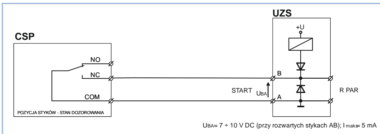
Rys. 15 Sterowanie wyjściem przekaźnikowym bezpotencjałowym (wariant 2).
