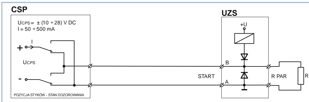
Rys. 16 Sterowanie wyjściem potencjałowym.
