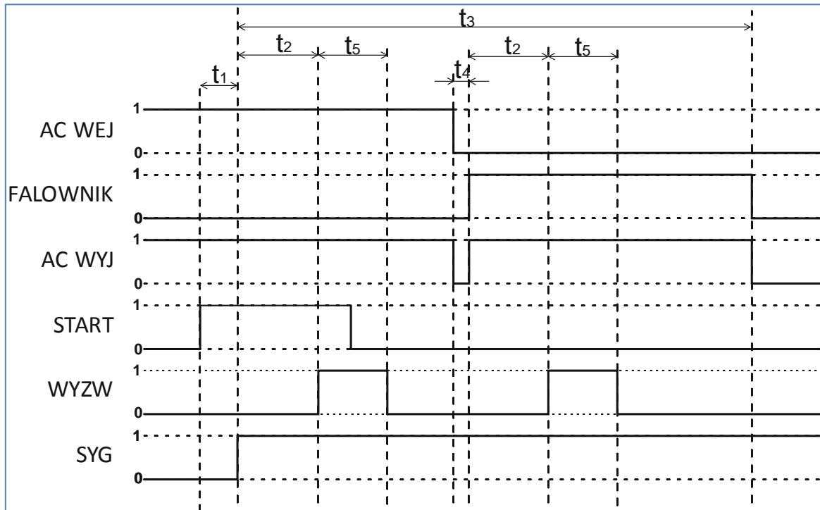
Rys. 6. Diagram pracy (przypadek 3).
