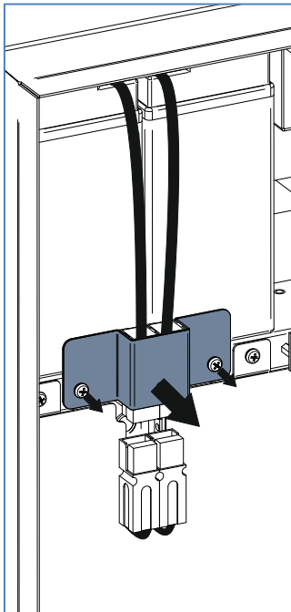
Rys. 22. Demontaż uchwyty baterii.
