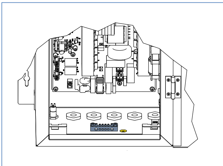
Rys. 17. Punkt zbiorczy uziemienia.
