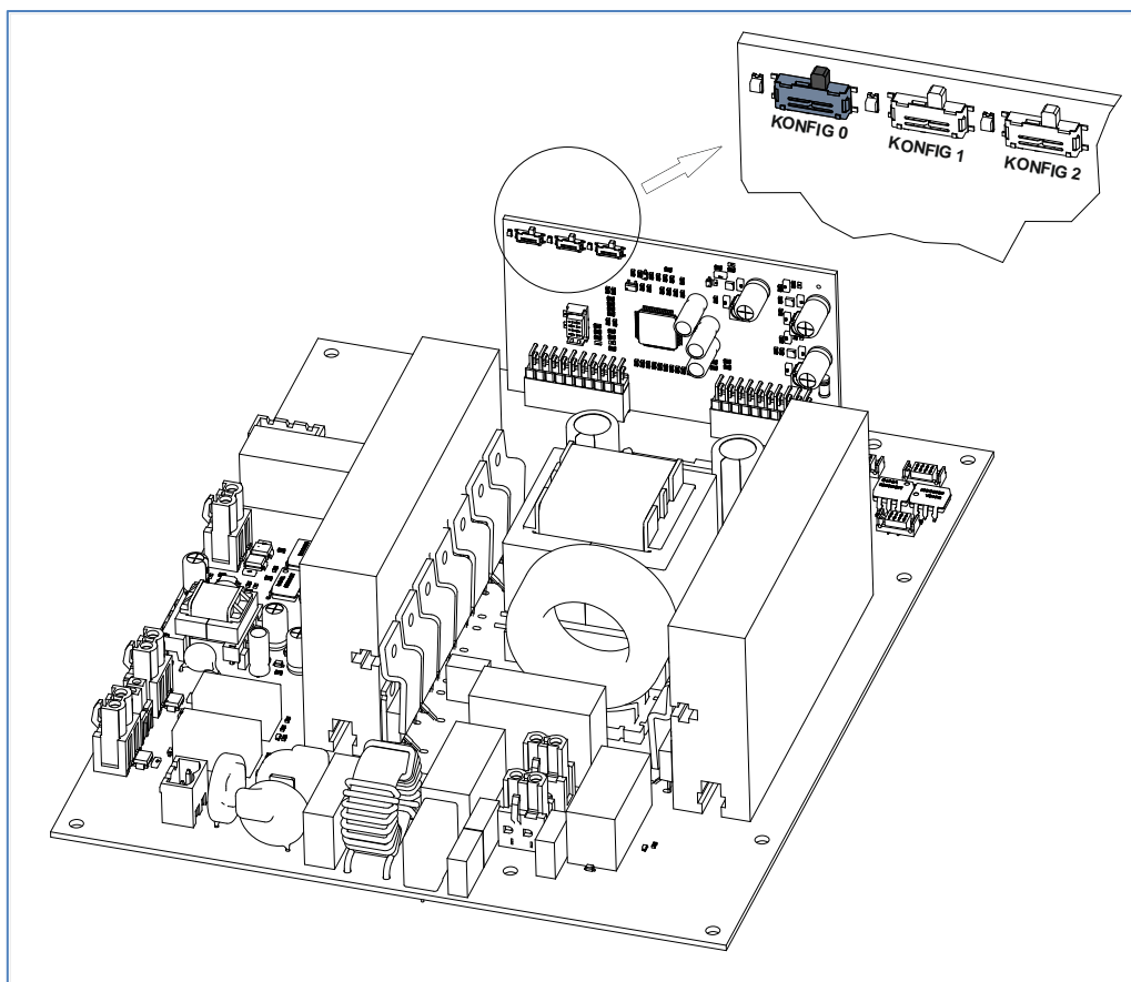
Rys. 19. Widok przełączników konfiguracyjnych.
