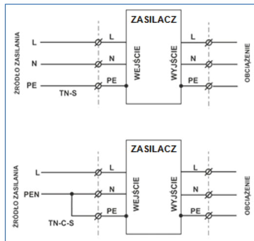
Rys. 8 Instalacja wejściowa zasilacza
