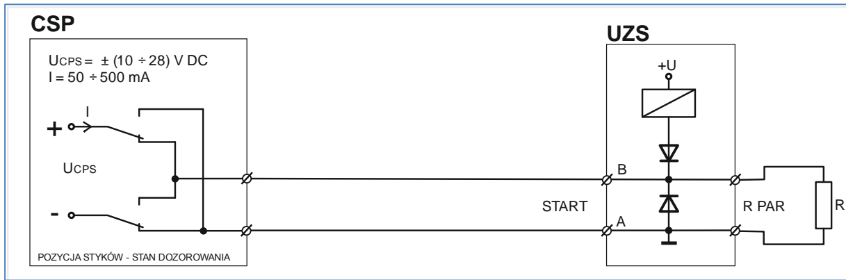
Rys. 17 Sterowanie wyjściem potencjałowym.
